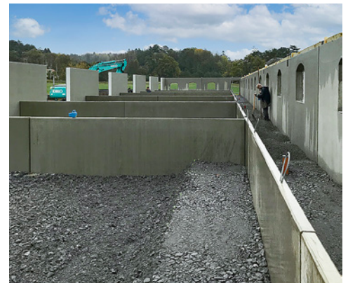
Montage av grisinnervägg (standardelement).
